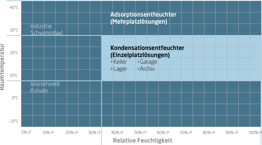
Arbeitsbereich Adsorptionsentfeuchter
