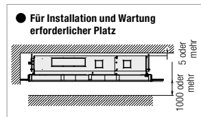
Dimension Ablauf-Steigrohr
