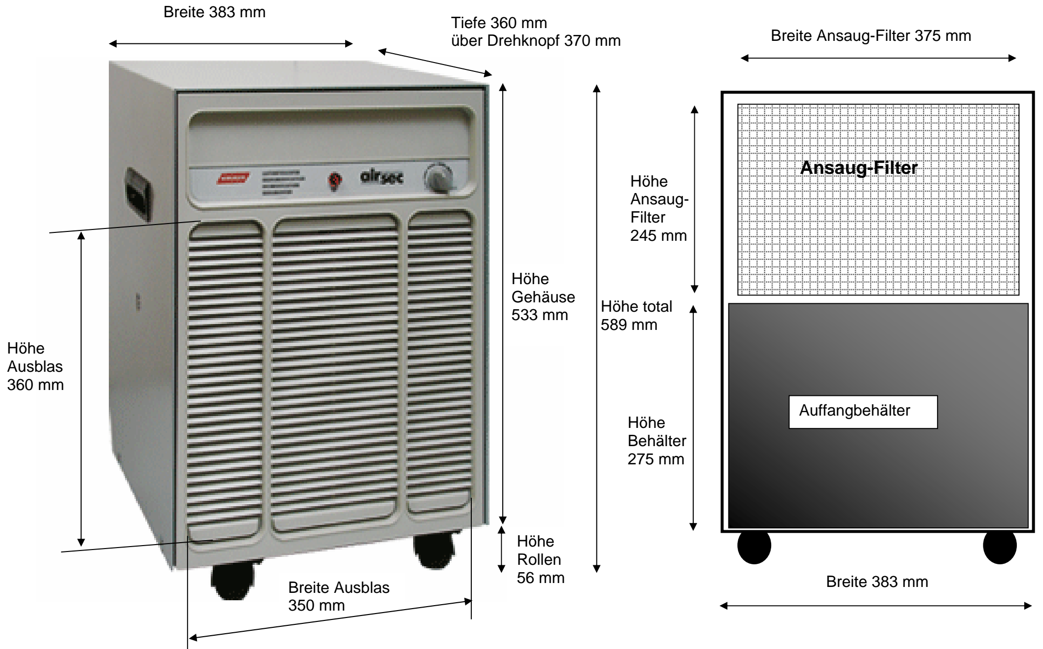
Ansicht hinten
