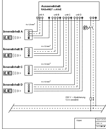
Anschlusschema für 4-Raum-Multi-Split Inverter-Modelle
