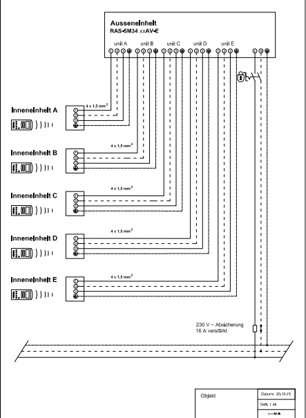
Anschlusschema für 5-Raum-Multi-Split Inverter-Modell
