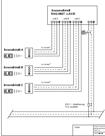
Anschlusschema für 3-Raum-Multi-Split Inverter-Modelle
