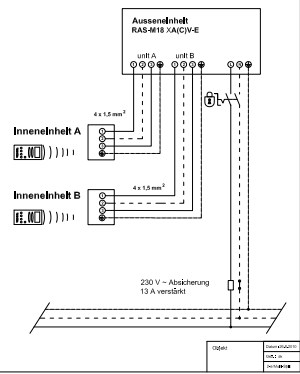
Anschlusschema für 2-Raum-Multi-Split Inverter-Modelle
