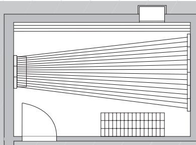
Sistema di stenditoio a cordine Sun-Line montaggio da parete a parete
